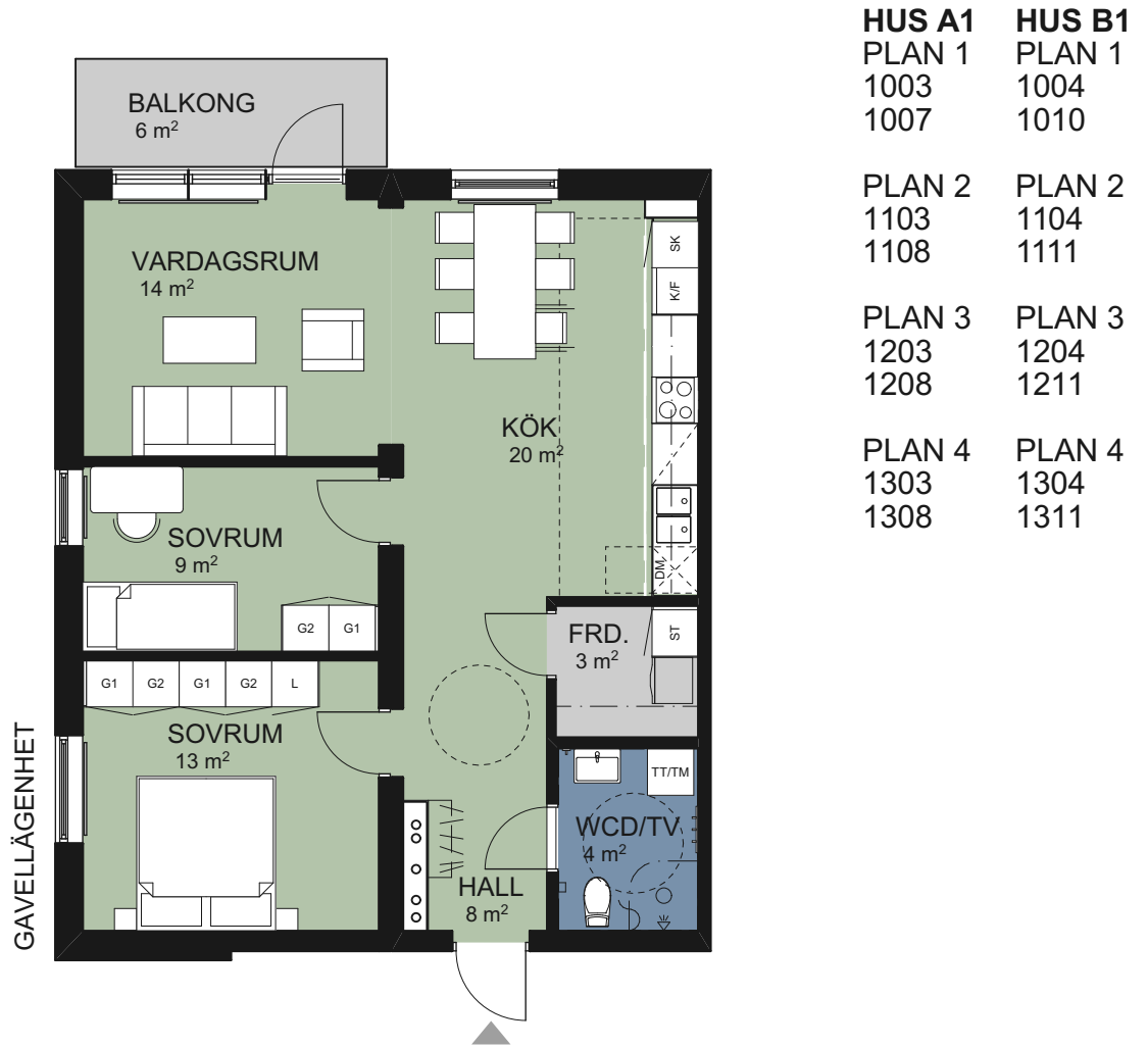
LÄGENHET 3 RoK BOA: 74,8 kvm
